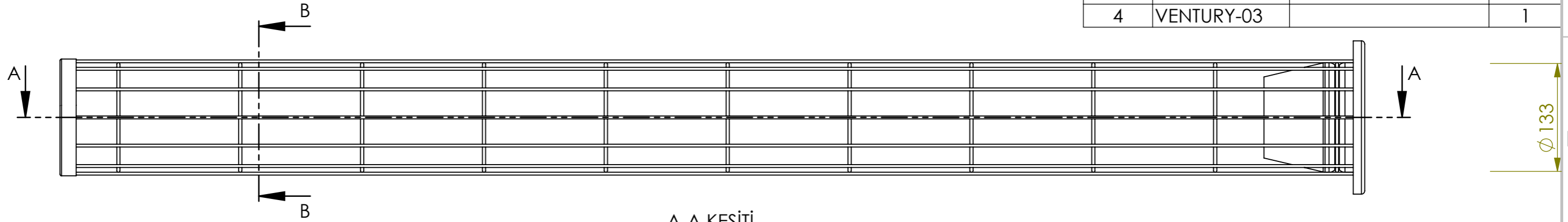
A-A KESİTİ (1 : 5)
