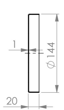
E-E KESİTİ (1 : 4)
